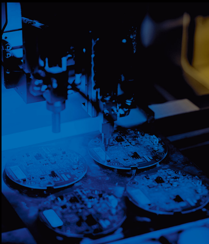
Automaty do lakierowania (PVA Delta 6 oraz Delta 8), mycia (Compa Clean III), testowania (AOI) oraz depanelizacji paneli PCB (Schunk SAR1300)
